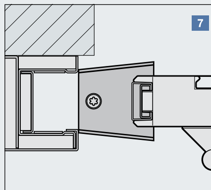
Οδηγός πόρτας με πέλμα εισόδου (σε πόρτες από 20 m 2 επιφάνεια πόρτας)
