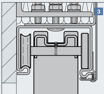
Ακριβής οδηγός φύλλων με ασύμμετρο γεωμετρικό οδηγό
