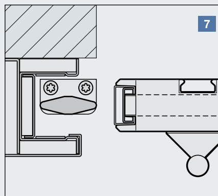
Οδηγός πόρτας με εγκατεστημένο στο δάπεδο κεντράρισμα εισόδου (σε πόρτες από 20 m 2 επιφάνεια πόρτας)
