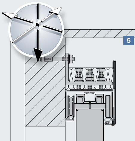
Απλή συναρμολόγηση χάρη στην τρισιδιάστατη ευθυγράμμιση
